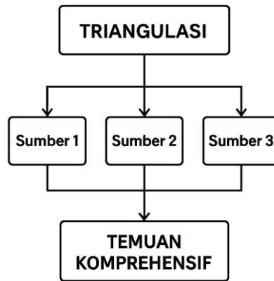
Gambar 1. Metode Triangulasi
