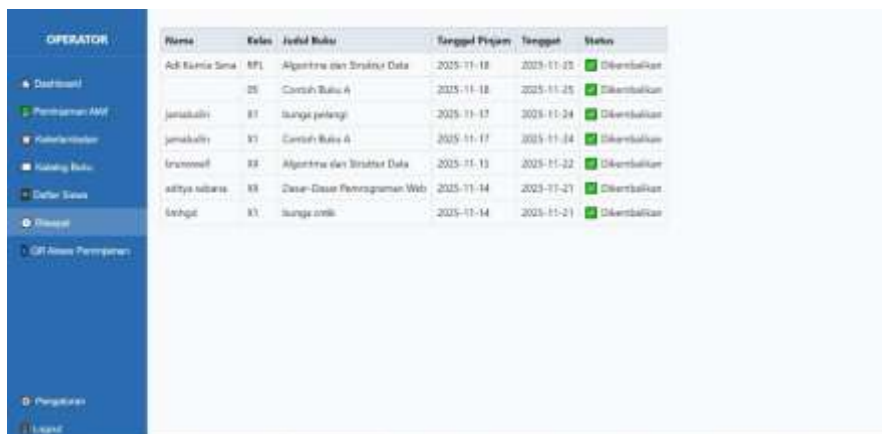
Gambar 4.4.8.1. Tampilan fitur riwayat
