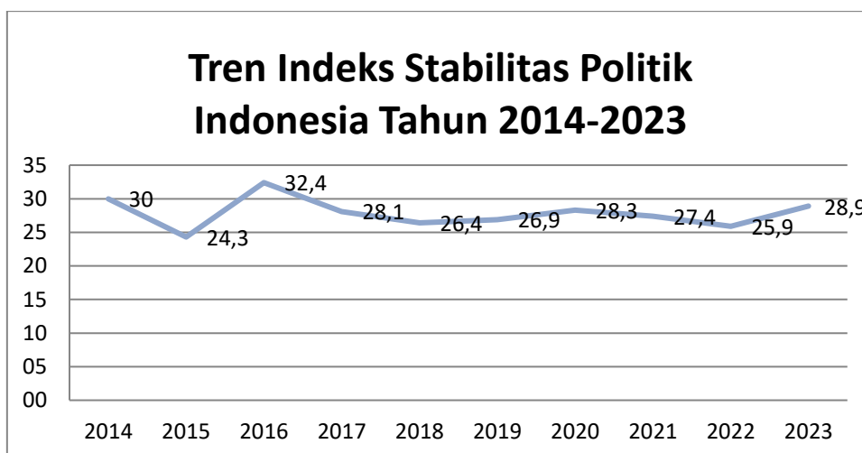
Grafik 1. Tren Indeks Stabilitas Politik Indonesia Tahun 2014-2023
